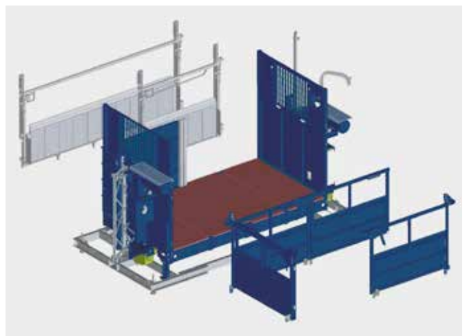
Mulige utvidelser av grunnenhet med to master (MX 1524 / MX 2024) som lasteplattform på tvers (B-variant)
