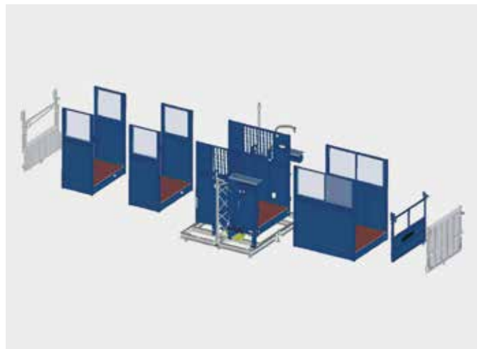
Mulige utvidelser av grunnenhet med to master (MX 1524 / MX 2024) som lasteplattform med gjennomgang (A-variant)
